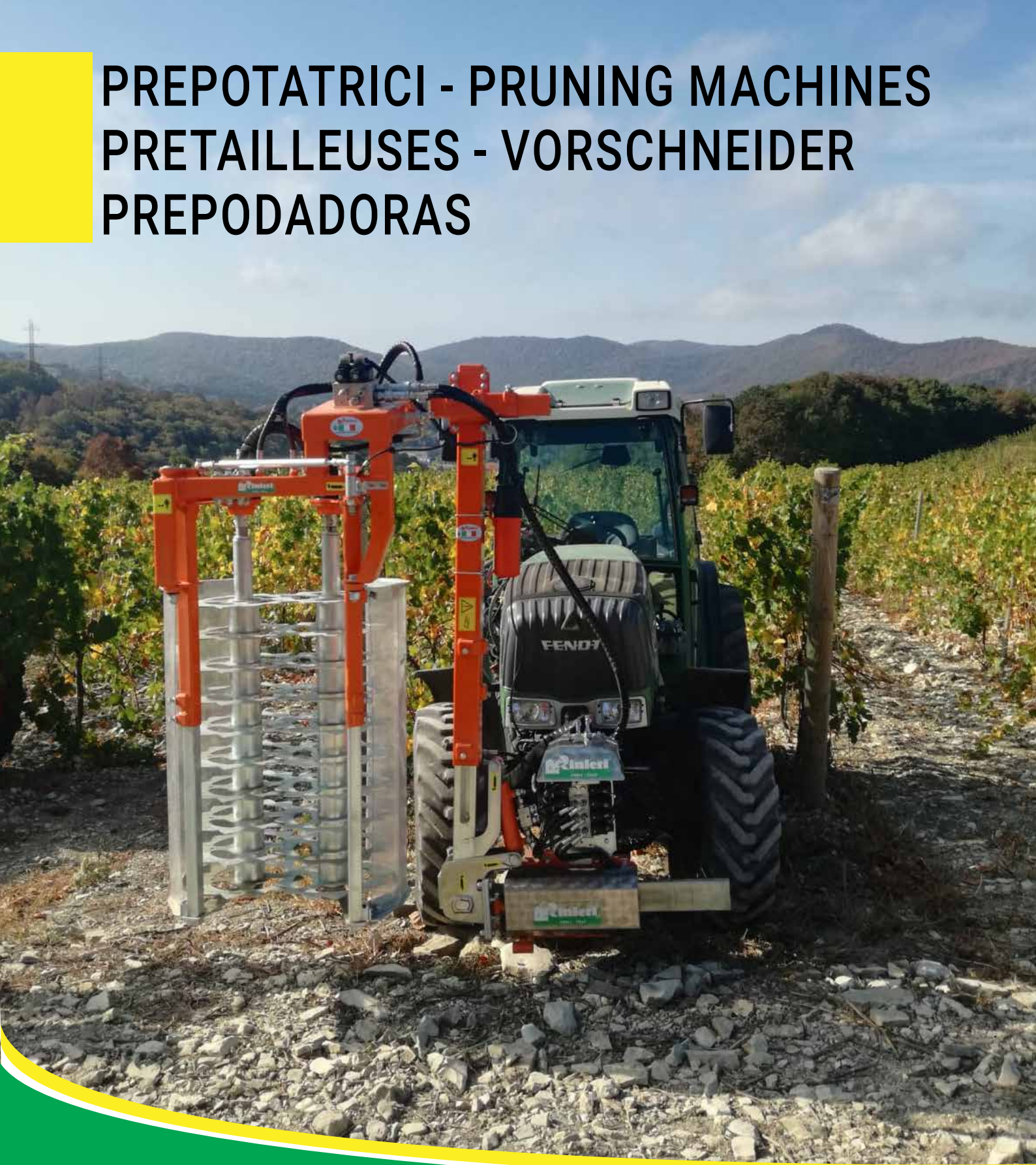
CPL VISION 1 PLUS - PRE-POTATRICE SU TELAIO VISION PLUS - PRE-PRUNING MACHINE ON VISION PLUS FRAME - PRETAILLEUSE SUR CHÂSSIS VISION PLUS - VORSCHNEIDER AN RAHMEN VISION PLUS - PRE-PODADORA EN CHASIS VISION PLUS
