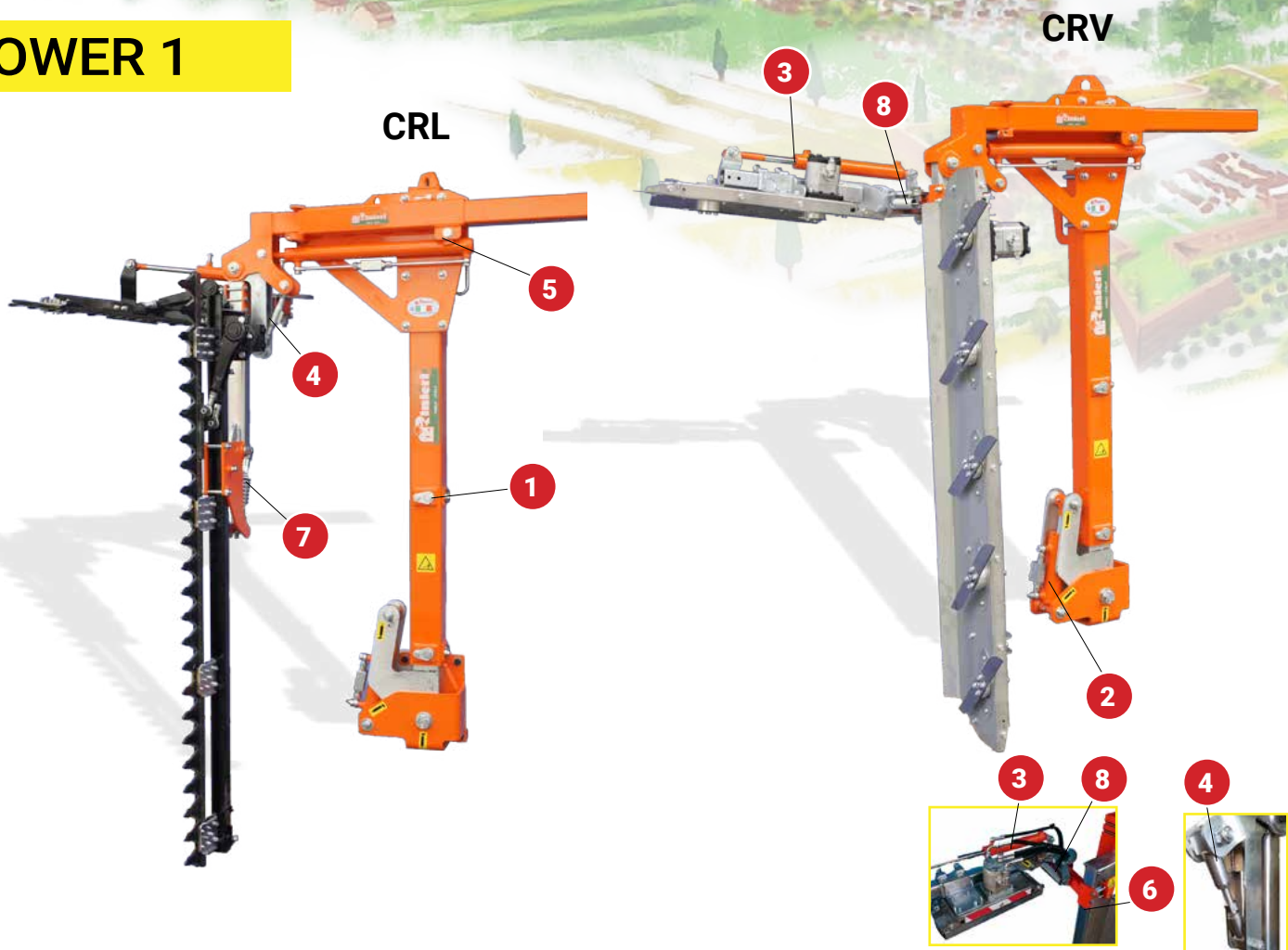
CIMATRICE SINGOLA TELAIO TOWER CON BARRE BILAMA O COLTELLI ROTANTI - SINGLE TOWER FRAME TRIMMER WITH DOUBLE SICKLE BAR OR BLADES - ÉCIMEUSE SIMPLE AVEC CHÂSSIS TOWER ET BARRES BILAMES OU COUTEAUX - EINSEITIGER LAUBSCHNEIDER AN RAHMEN TOWER MIT DOPPELMESSERSCHNEIDWERK ODER ROTIERENDEN MESSERN - DESPUNTADORA MODELO TOWER DE DOBLE SIERRA O CUCHILLAS ROTATIVAS
