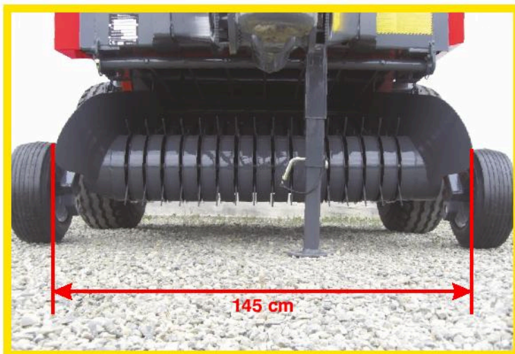
Raccoglitore di larghezza massima 145 cm. Pick-up max width 145 cm.
